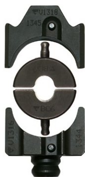
Outer die holder V1318, BC dies, inner die holder V1316.
